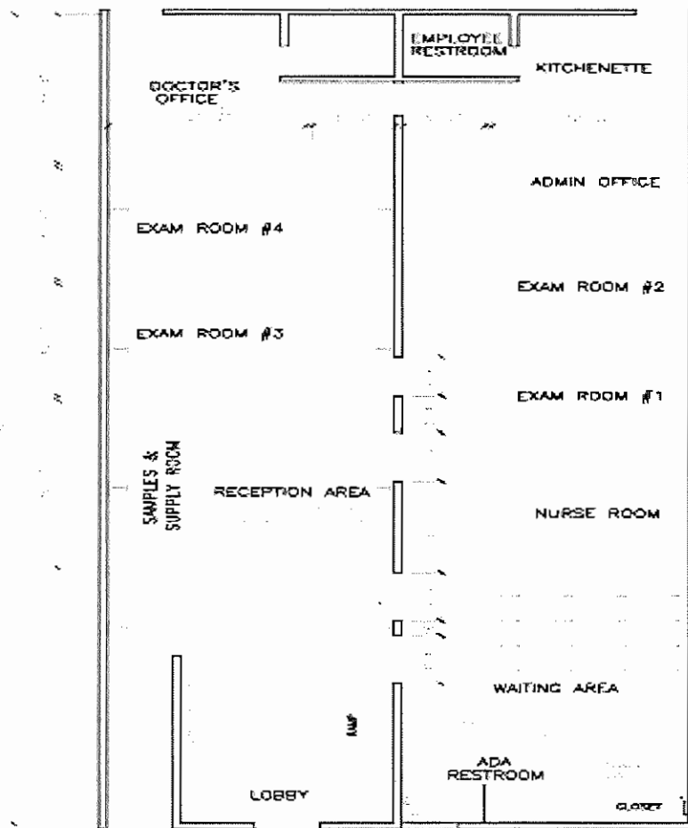
PLANTA DE PISO (PROPUESTA)
